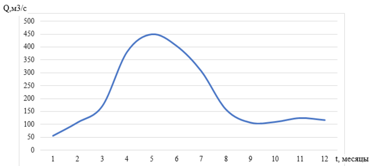
Рисунок 3.4. - Годовая кривая стока реки Кафирниган
