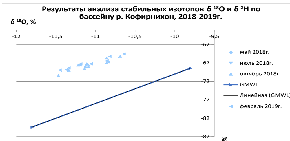
Рисунок 3.7. - Результаты исследования стабильных изотопов по р. Кофирниган (2018-2019 годы)
