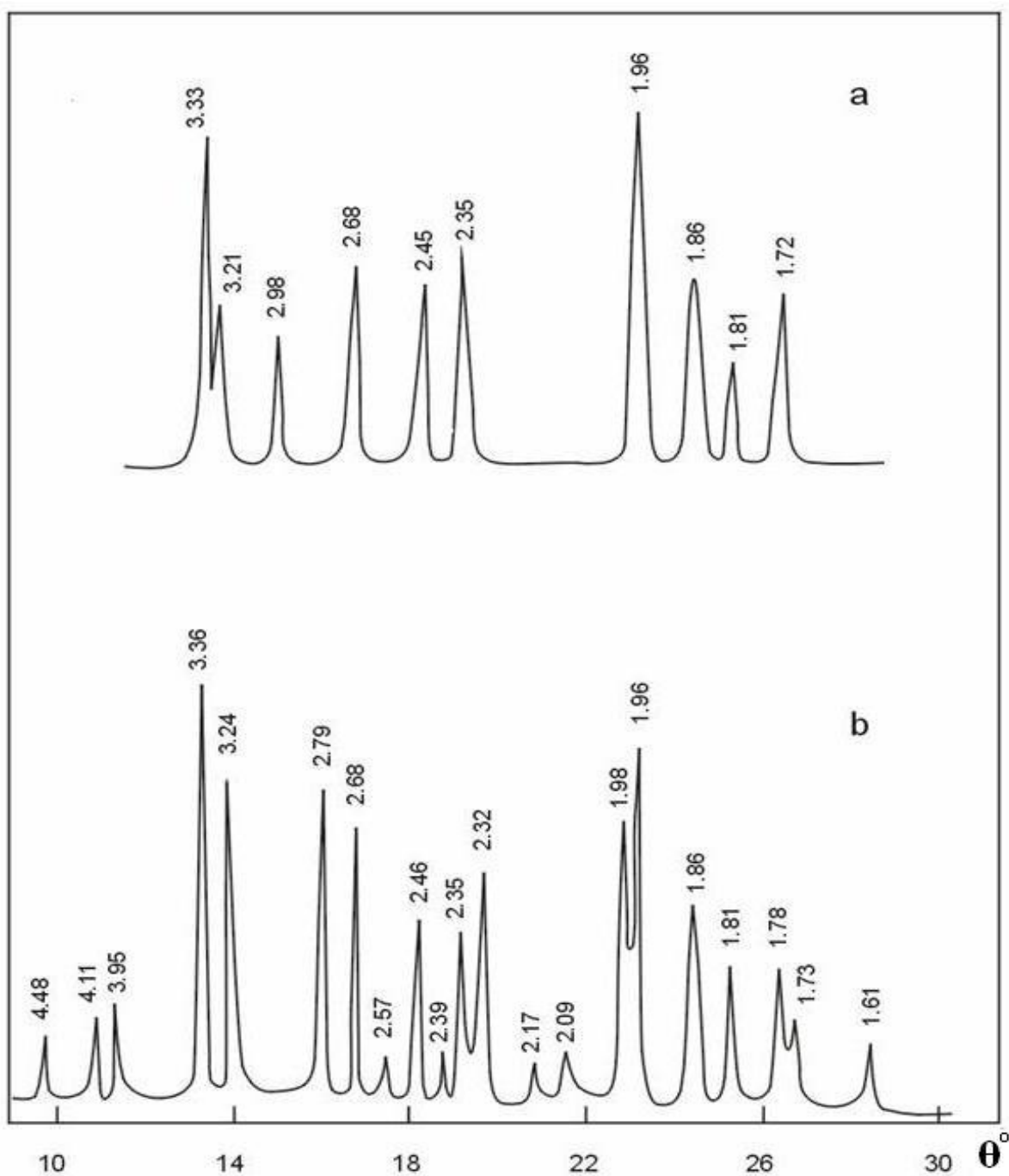
Рисунок 4.3. - Рентгенограмма осадков воды источников Момирак (а) и Тебалай (b).
