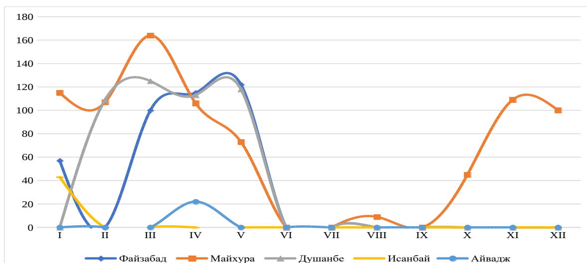
Рисунок 3.3. - Среднемесячное распределение осадков в зависимости от различной высотной зоны бассейна р. Кафирниган
