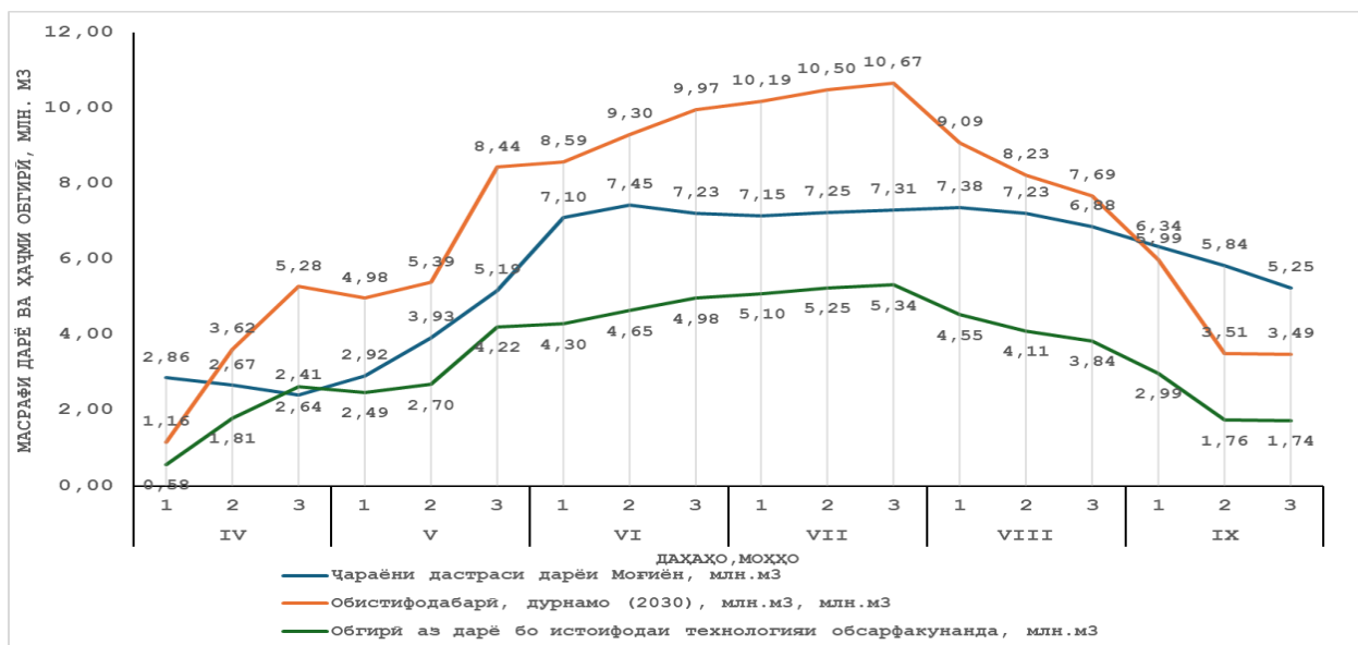
Расми 3.5. - Муқоисаи рёҷаи гидрологӣ дарёи Моғиён дар солҳои хушсолӣ бо назардошти обистиғодабарии дурнамо (2030) ва рёҷаи обғирӣ аз ин дарё бо назардошти ҷараёни талаботи экологӣ [4-М]
