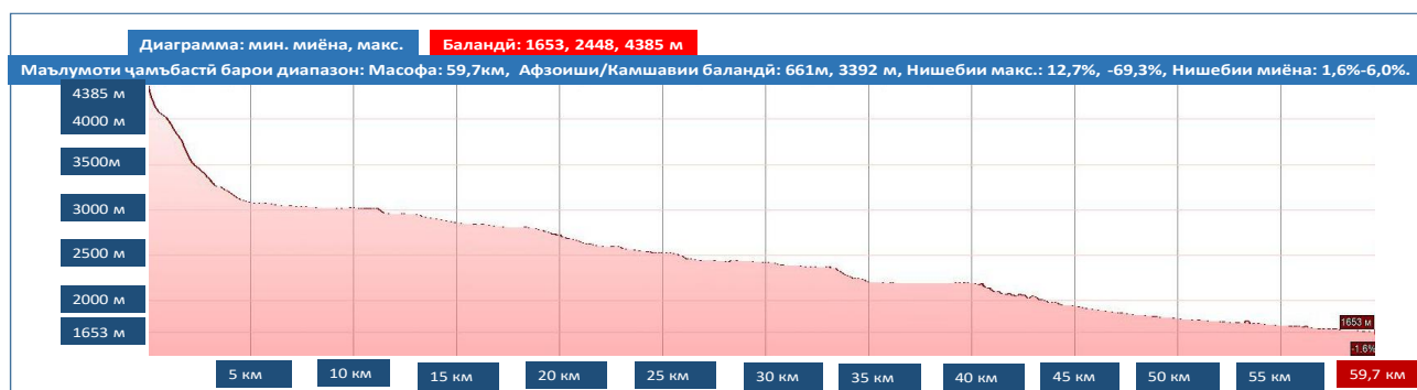
Расми 2.7. - Буриши тӯлии Искандардарё
