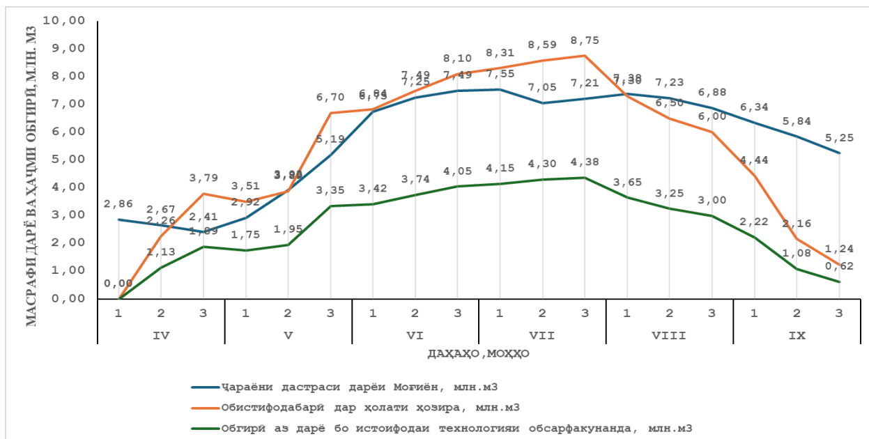
Расми 3.4. - Муқоисаи рёҷаи гидрологӣ дарёи Моғиён дар солҳои хушсолӣ ва рёҷаи обғирӣ аз ин дарё бо назардошти ҷараёни талаботи экологӣ [4-М]
