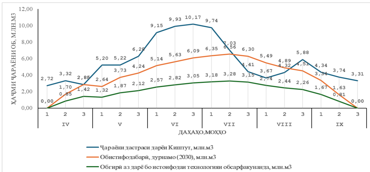
Расми 3.3 - Муқоисаи реҷаи гидрологии дарёи Киштуд дар солҳои хушксолӣ бо назардошти обистифодабарии дурнамо (2030) ва реҷаи обгирӣ аз ин дарё бо назардошти чараёни талаботи экологӣ [4-М, с. 168]
