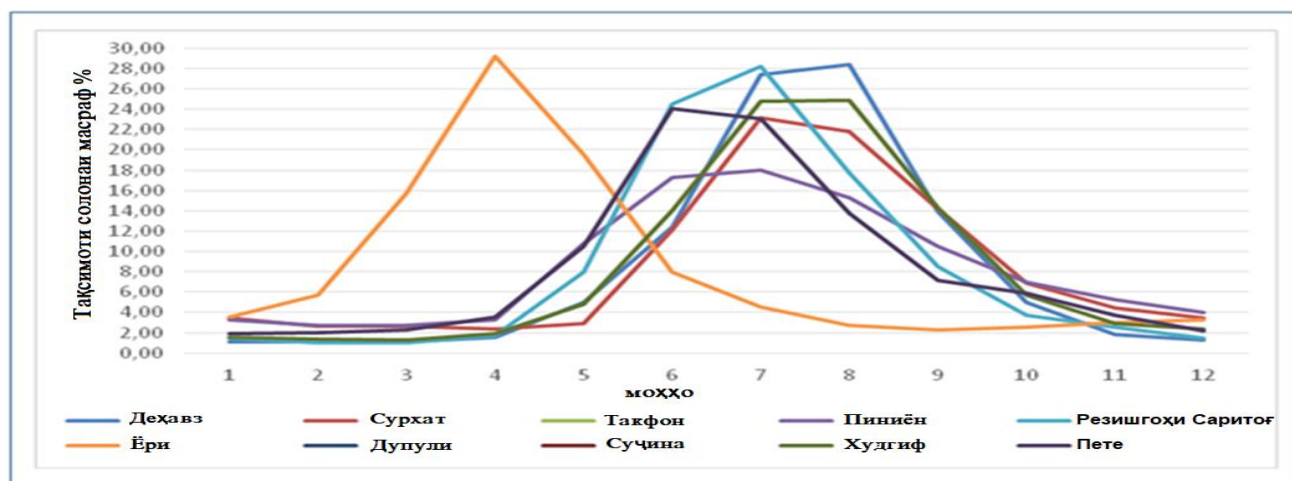
Расми 2.19. - Тақсмоти солонаи масрафи миёнаи моҳонаи об дар дидбонгоҳи гидрометрии ҳавзаи дарёи Зарафшон
