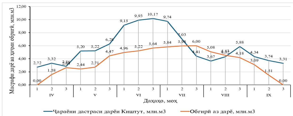
Расми 3.2 - Муқоисаи рёҷаи гидрологии дарёи Киштуд дар солҳои хушксолӣ ва рёҷаи обгирӣ аз ин дарё бо назардошти ҷараёни талаботи экологӣ [4-М, с. 168]
