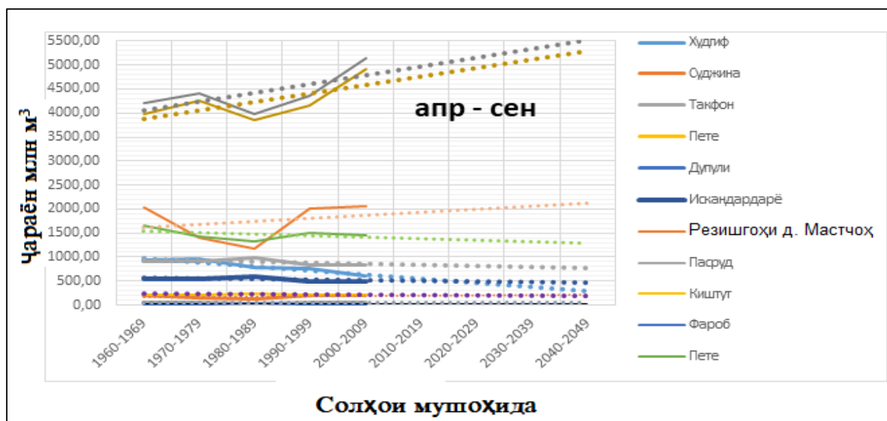
Расми 2.18 - Ҷараёни миёнаи бисёрсолаи оби дарё дар фаслҳои сол, аз моҳи апрел то сентябр, аз соли 1960 то соли 2010
