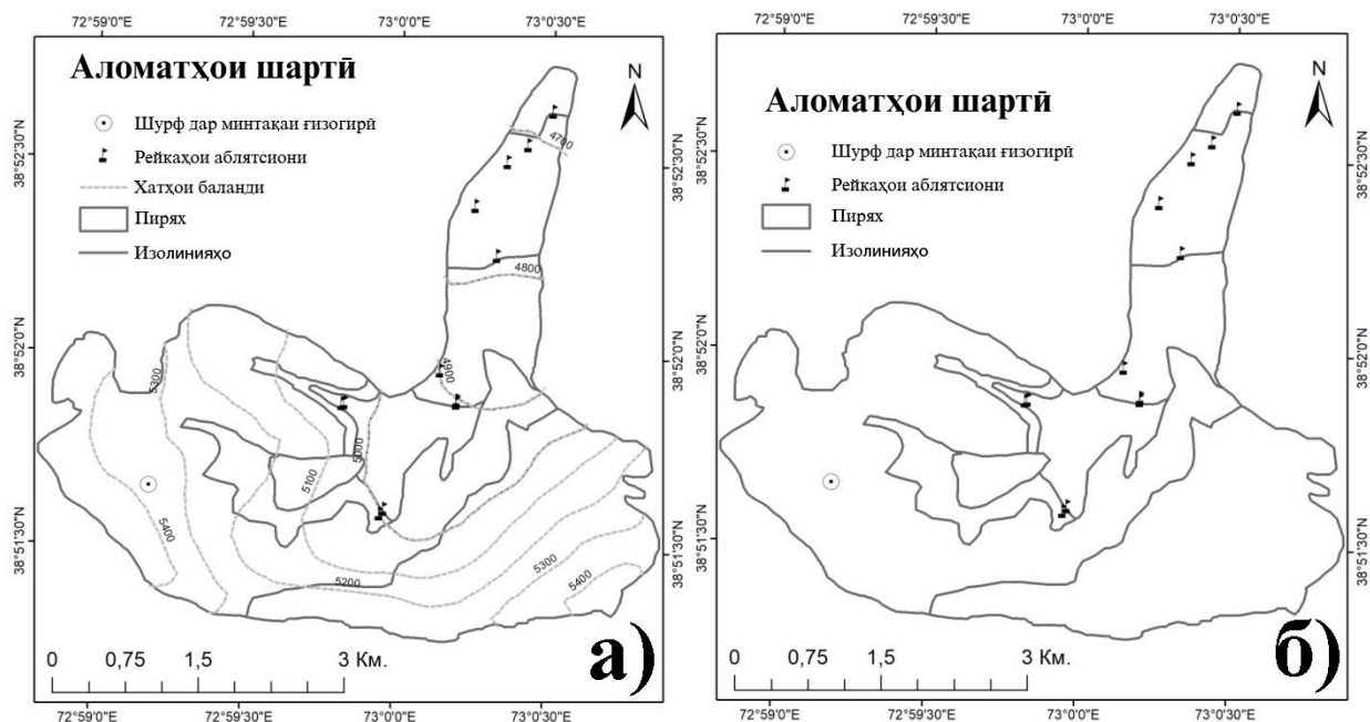
Расми 2. – Муайян намудани тавозуни ҳаҷми пириях. Усули профилӣ (а), усули изолиния (б)
