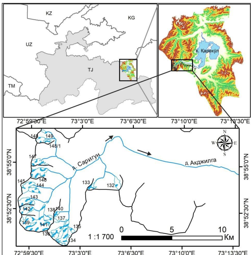
Расми 3. - Ҳавзаи дарёи Саригун, шоҳоби кӯли Ховаркӯл (Таҳиягар муаллиф)
