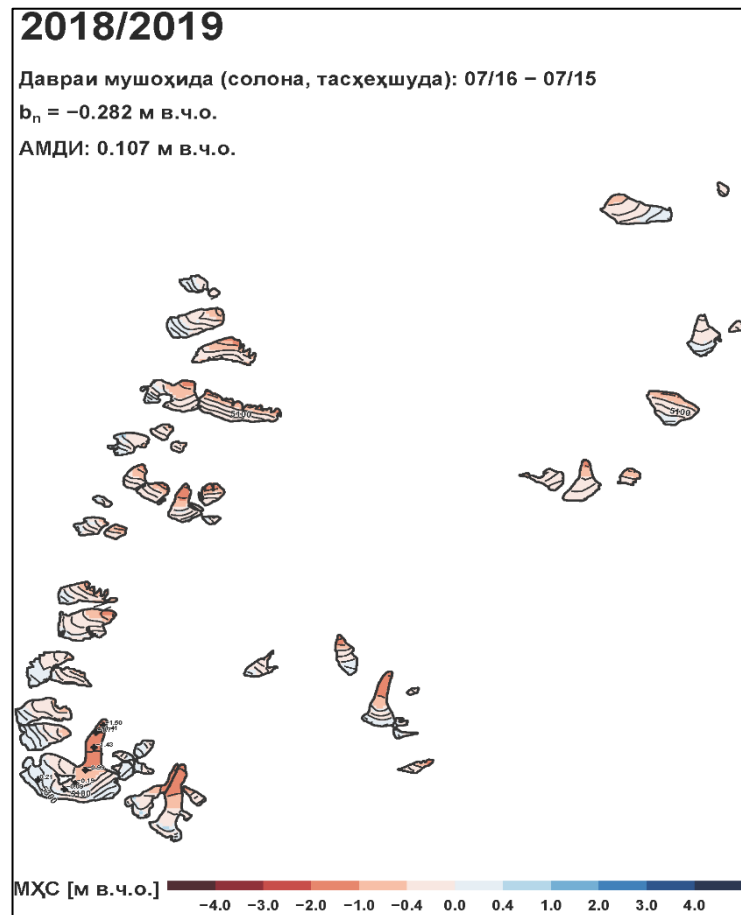
Расми 9. - Амсиласозии тавозуни ҳаҷми пирахҳо дар ҳавзаи дарёи Саригун, шоҳоби кӯли Ховаркӯл
