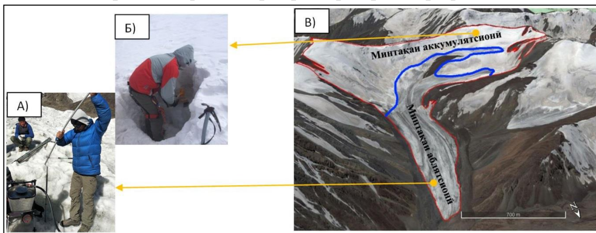
Расми 1. - Усулҳои асосии корҳои сахроӣ: А) Рейка дар минтақаи аблятсионӣ; Б) Чох дар минтақаи аккумулятсия; Б') Минтақаҳои аблятсия ва аккумулятсияи пириях
