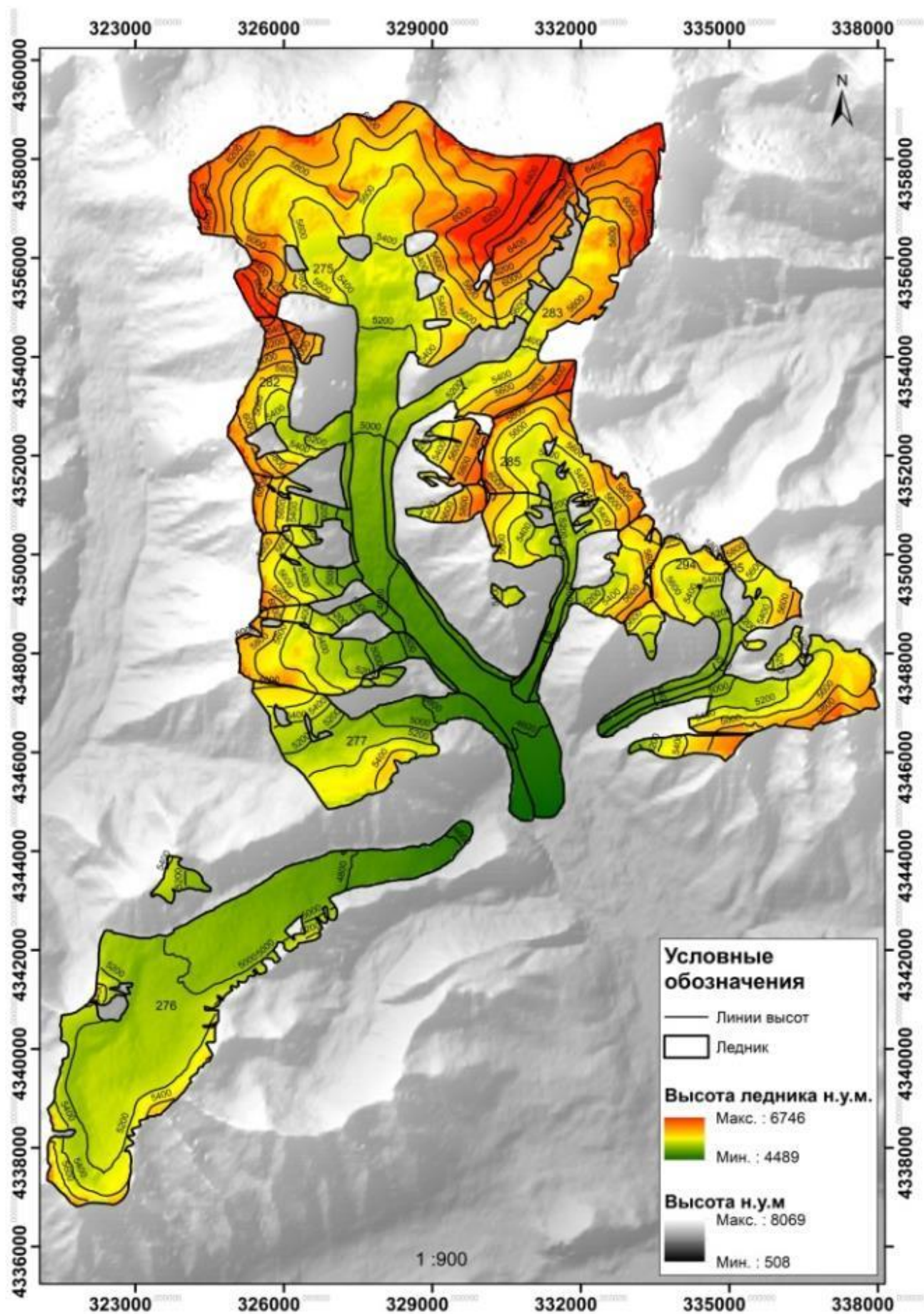
Рисунок 3.3. – Ледник Октябрьский
