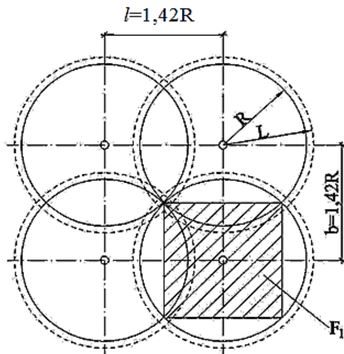
Рисунок 4.7. Принятая схема расположения дождевальных аппаратов R -расчетный радиус действия дождевателя, м; L -дальность полета струи, м; F -площадь полива с одной стоянки, m^2 .
