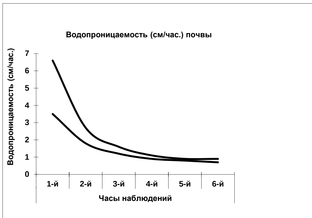
Рисунок 4.2. - Водопрооницаемость среднесуглинистых и тяжелосуглинистых почв Центрального Таджикистана
