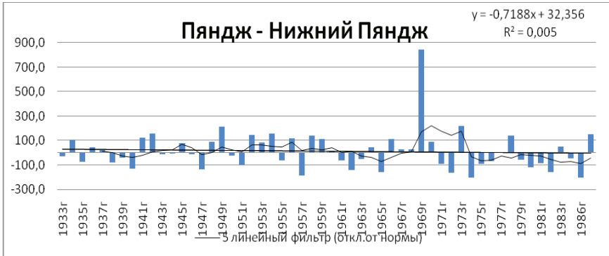
Рис. 4.10. Изменение расходов воды (м 3 /с) на р. Пяндж пост Нижний Пяндж за период наблюдений с 1933 по 1987гг.
