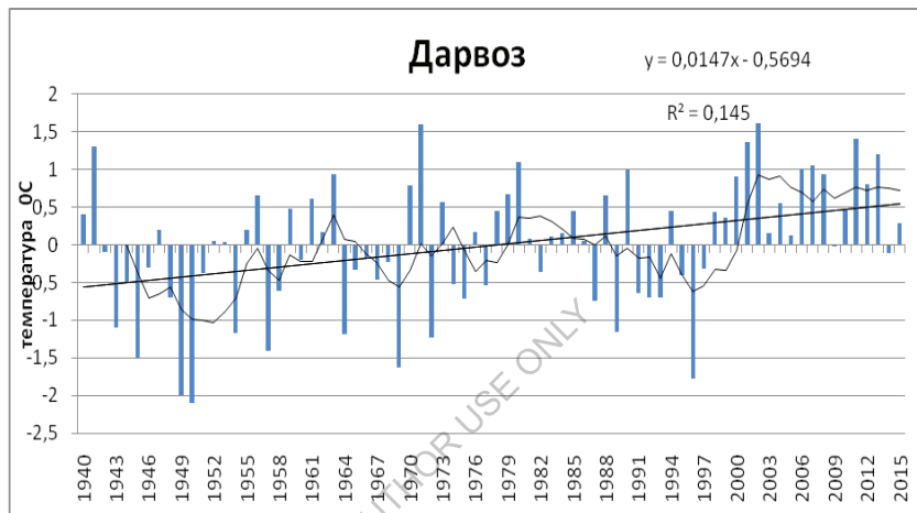
Рис. 3.11. Колебания температуры воздуха на территории Дарвоза.
