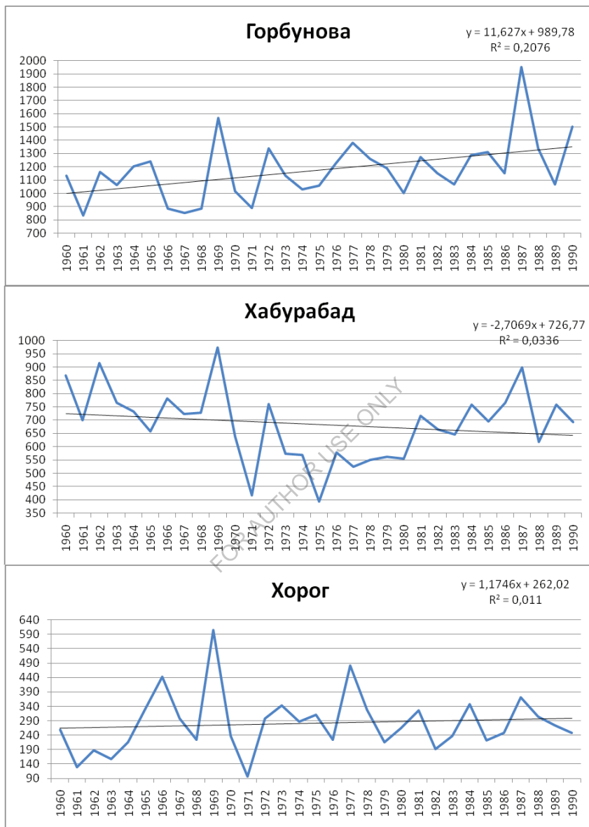
Рис. 3.7. Трендовый анализ изменения количества осадков на станциях им.Горбунова, Хабурбад, Хорог.
