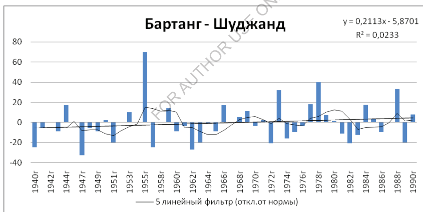
Рис. 4.12. Отклонение средних годовых расходов воды (м 3 /с) от среднего за базовый период на р. Бартанг пост Шуджанд за период наблюдений 1940-1990гг.
