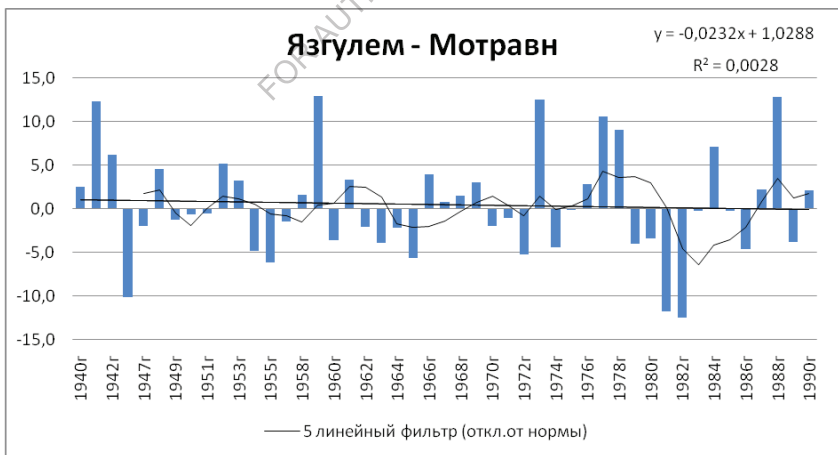
Рис. 4.11. Отклонение средних годовых расходов воды (м 3 /с) от среднего за базовый период на р. Язгулем пост Мотравн за период наблюдений 1940-1990гг.
