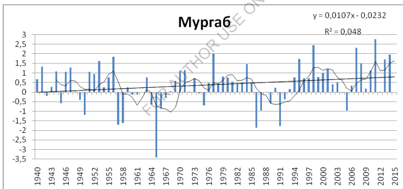
Рис. 2.6. Отклонение средней годовой температуры воздуха от нормы на территории Мургаба за 1940-2015 гг.
