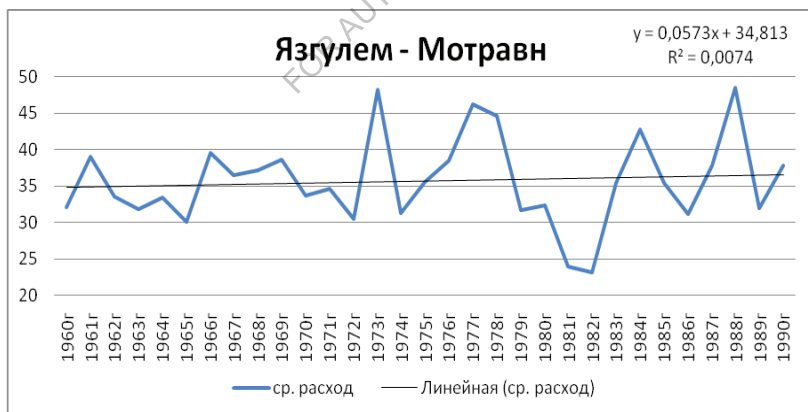
Рис. 4.6. Изменение расходов воды (м³/с) на р. Язгулем пост Мотравн за базовый период.
